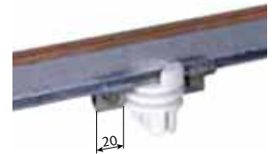
Abbildung zeigt einen Isolator mit 2 Sicherungsklemmen (Festpunkt).
